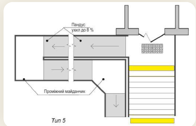
Рисунок 1.23.3. Типи облаштування вхідної групи (продовження): д) П-подібний пандус
